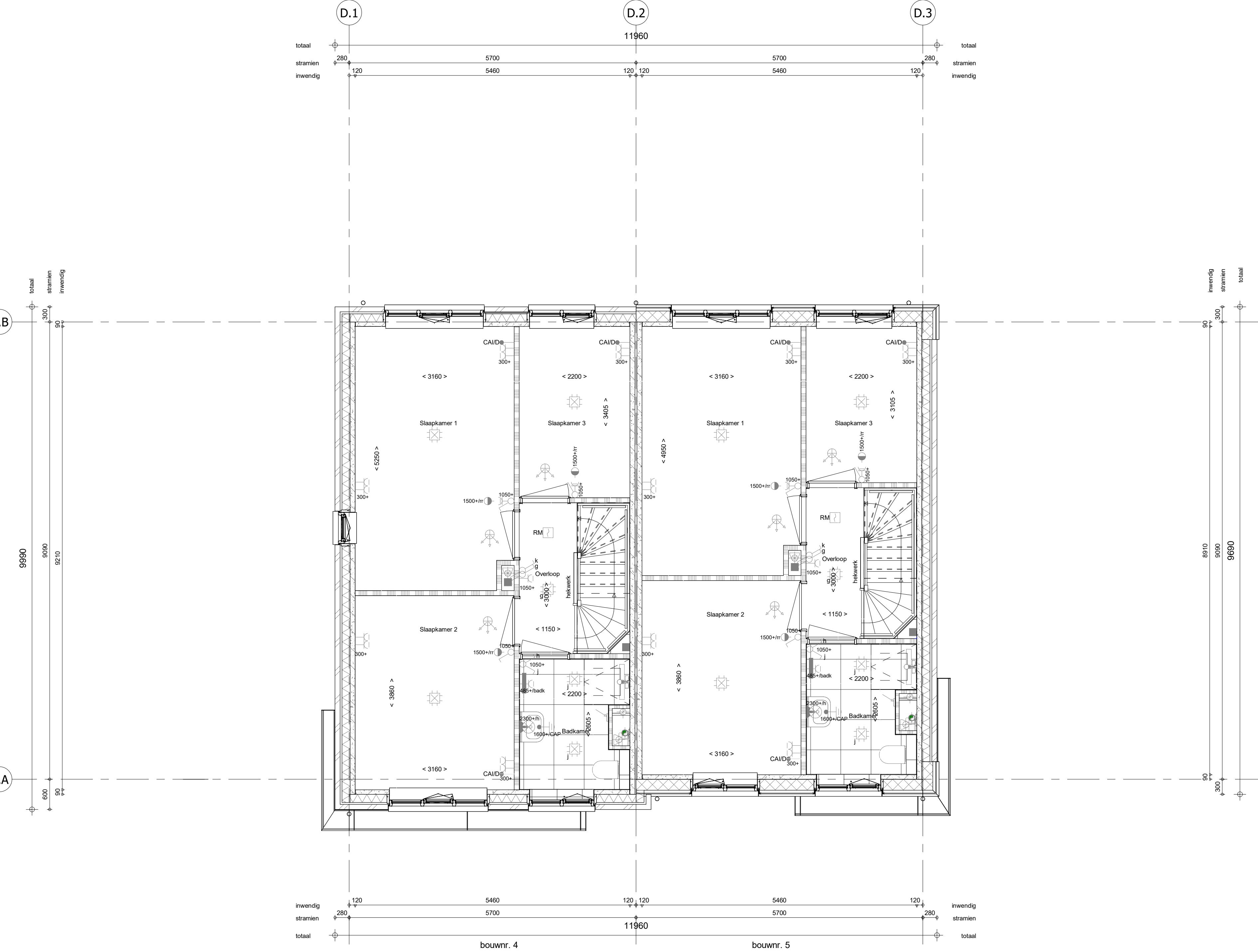
1e verdieping 1 : 50
