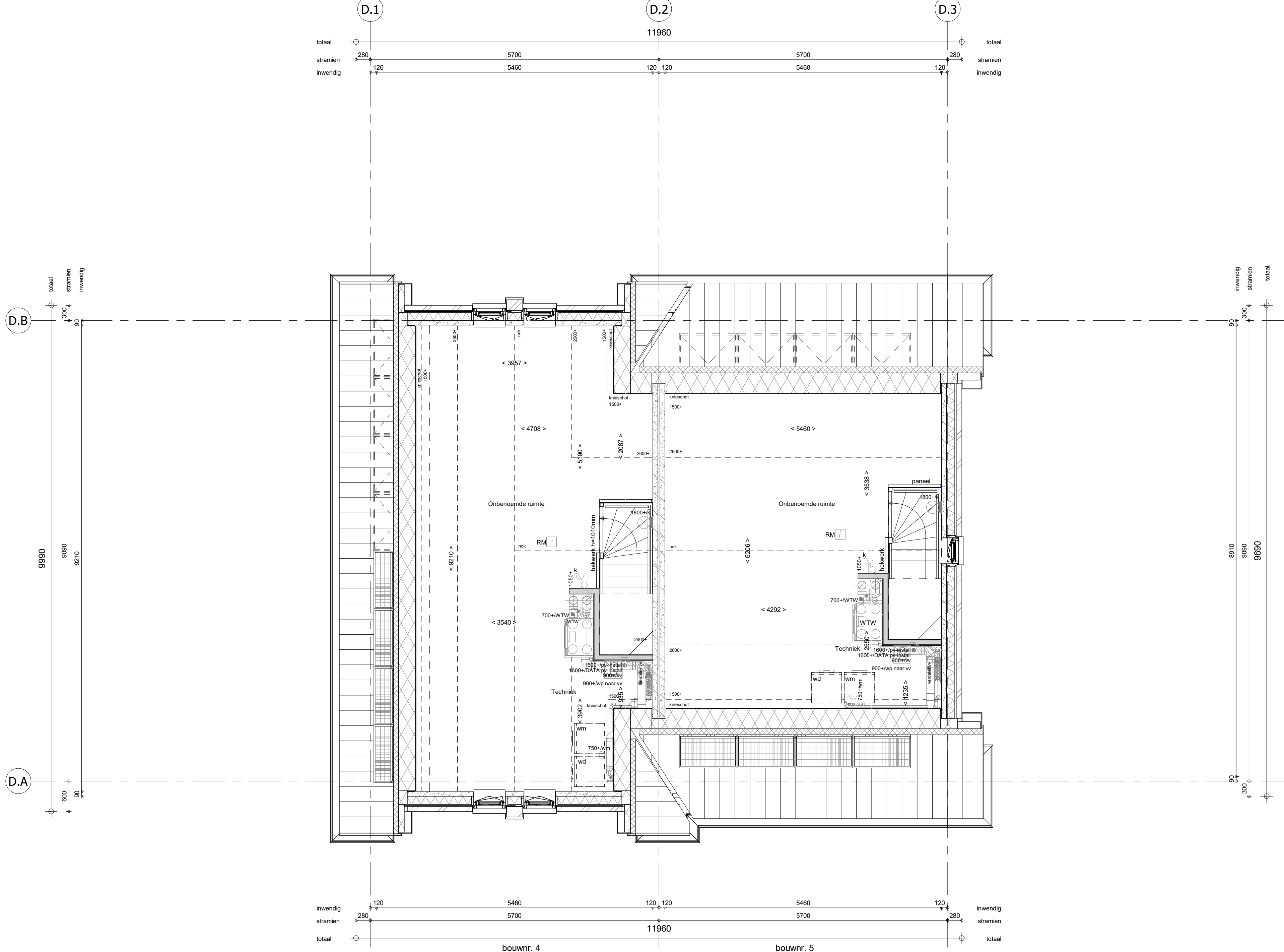
2e verdieping 1 : 50
