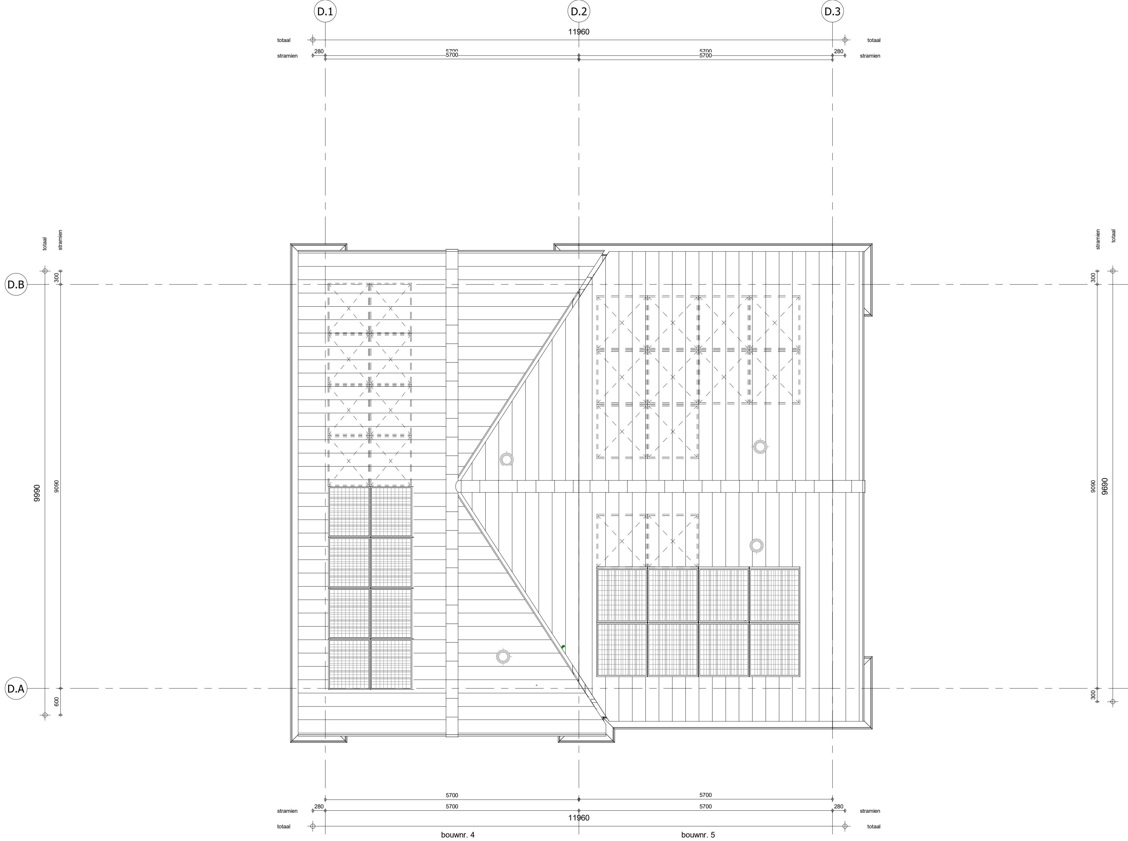
Dakaanzicht 1 : 50
