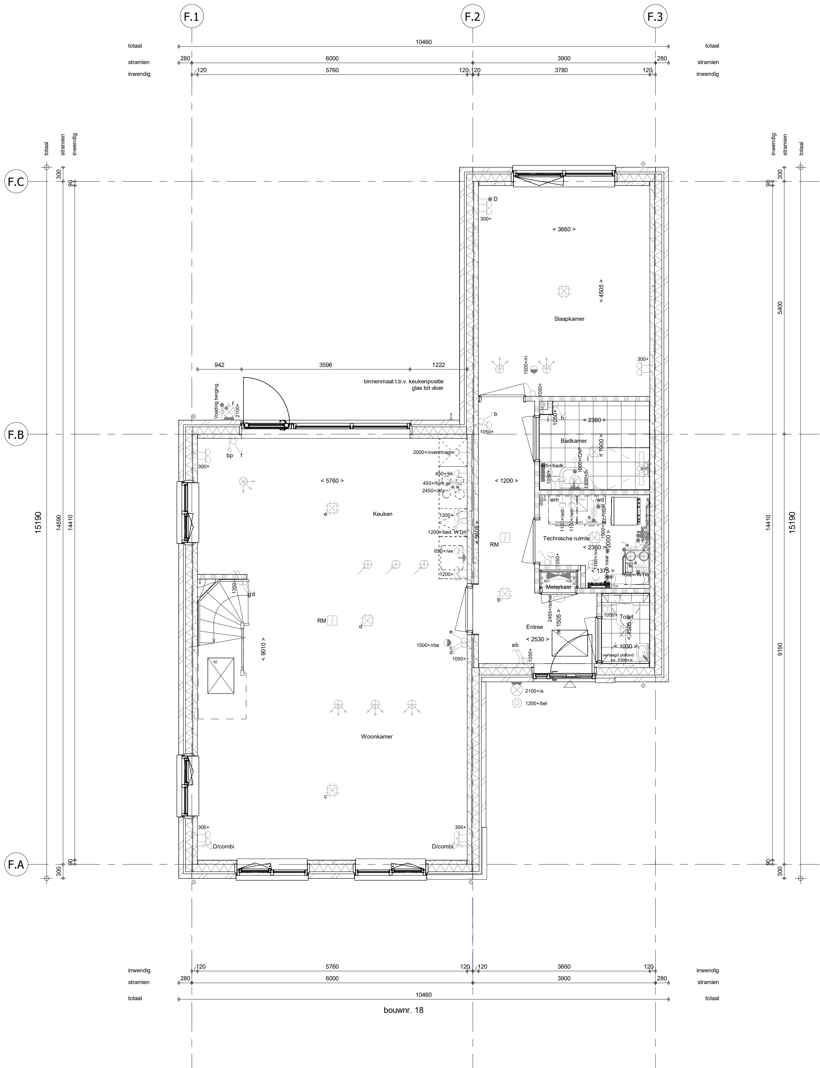
Begane grond 1 : 50
