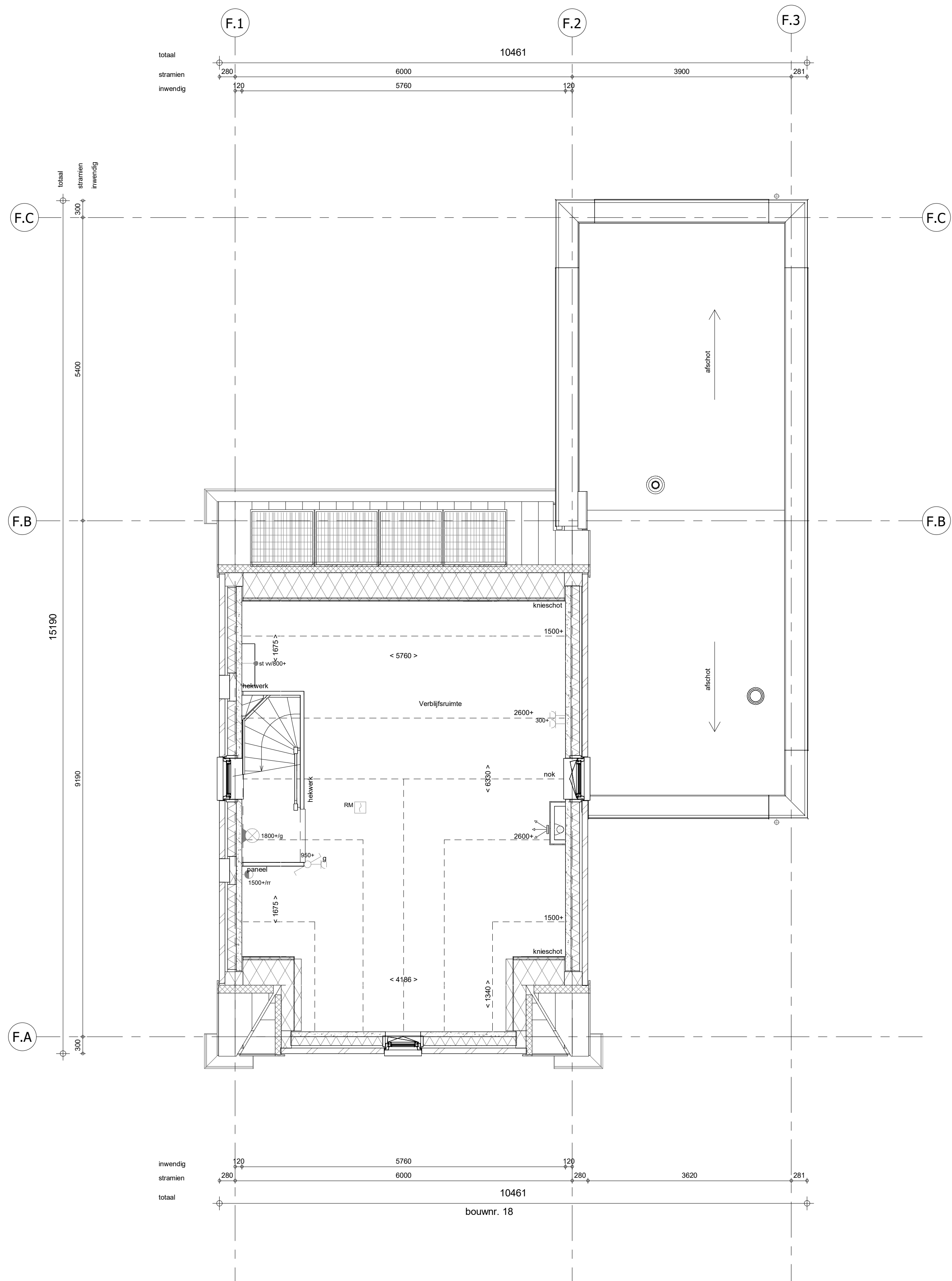
1e verdieping 1 : 50
