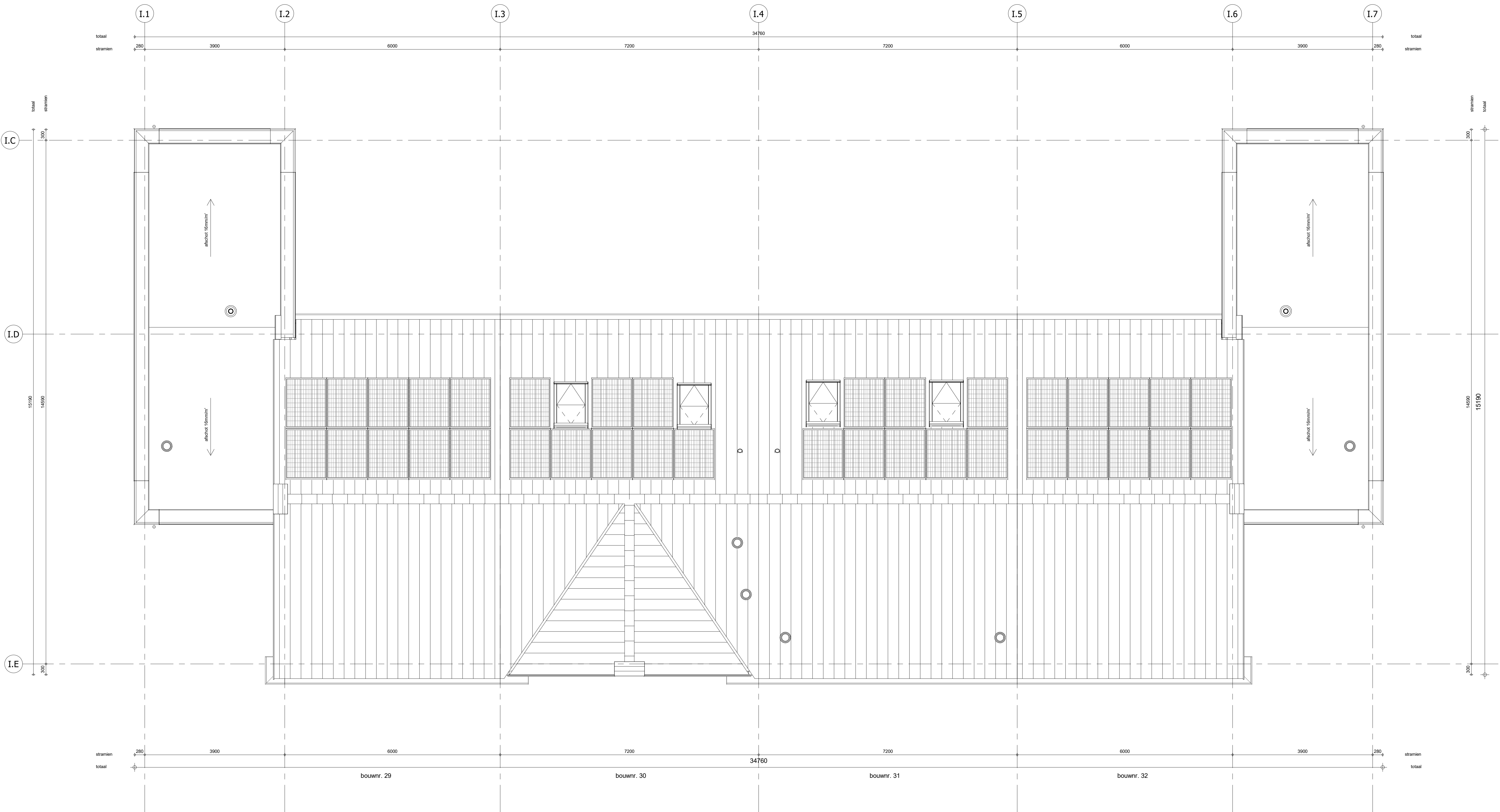
Dakaanzicht 1 : 50
