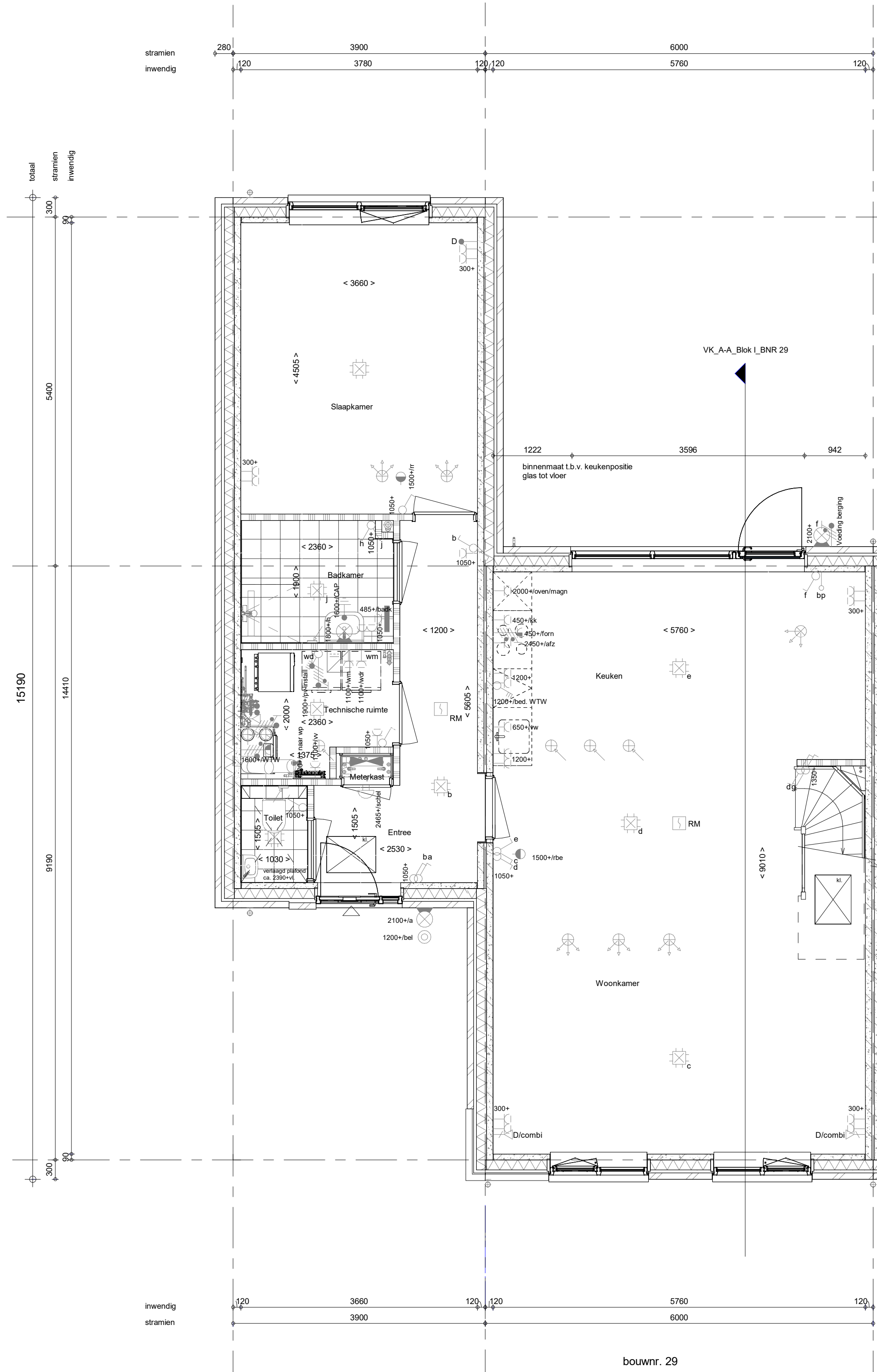
Begane grond 1 : 50
